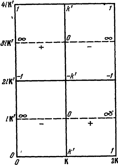
Рис. 5. \operatorname{dn}(u) для 0 \leq \operatorname{Re} u \leq 2K , 0 \leq \operatorname{Im} u \leq 4K' .
