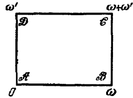
Рис. 11. z' -плоскость.
