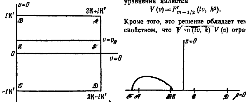
Рис. 15. Отображение (5).
