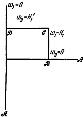
Рис. 12. Отображение w = \zeta(z) + e_1 z .
